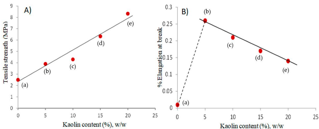
Рисунок 4 – Влияние содержания каолина на прочность при растяжении (А) и относительное удлинение (В) при разрыве пленок, полученных из (а) K0SNC, (b) K5SNC, (c) K10SNC, (d) K15SNC и (e) пленки K20SNC. KSNC: нанокompозит каолинового крахмала [20]
