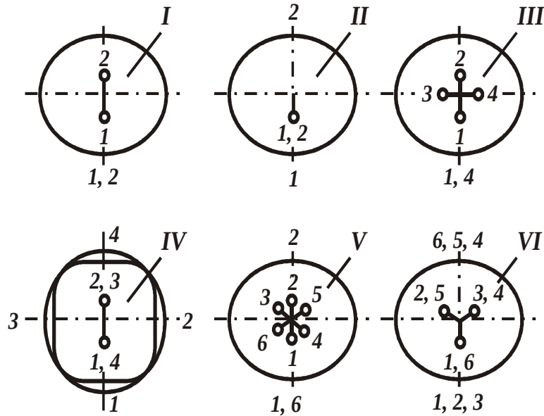
Рисунок 4 – Схема расположения эксцентриков в многороторных рабочих органах:
