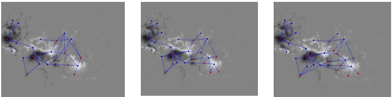
Рисунок 1 – Критические сети построенные для трех последовательных во времени магнитограмм АО
