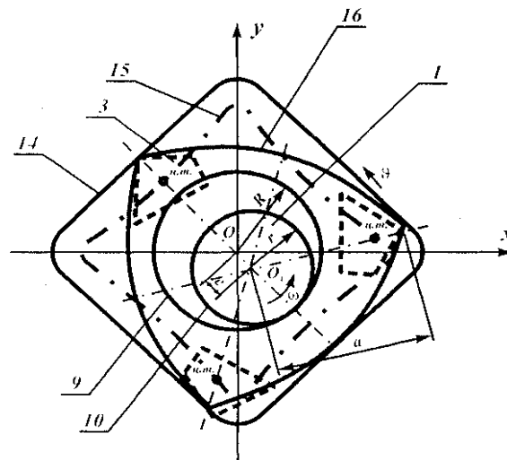
Рисунок 2 – Образование гипотрохоид
