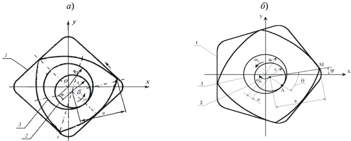
Рисунок 3 – Образование гипотроклоид а) с треугольной формой; б) с четырехугольной формой: 1 – гипотрохоида; 2 – сателлит; 3 – колесо зубчатое
