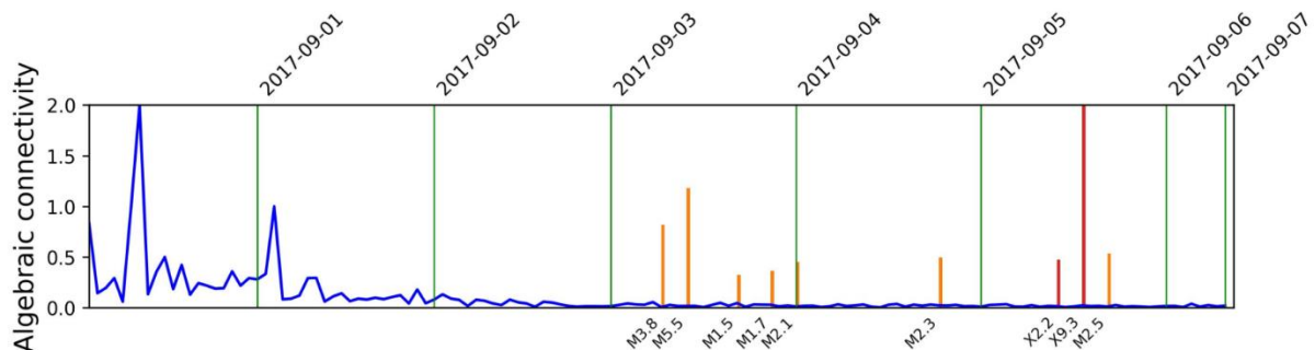
Рисунок 2 – Изменение \lambda_2 во времени для критических сетей АО. Вспышки показаны вертикальными барами
