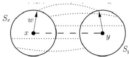
Рисунок 3 – Изменение кривизны для дуги, связывающей пару точек (x, y)
